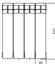
модель Base 350
